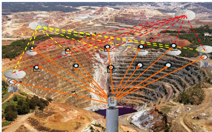
19 Сурет – Какарьердегі GPS құрылымдарының схемасы
