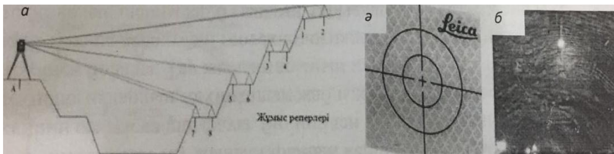
24 Сурет – Бақылау маркасы арқылы қадағалау
