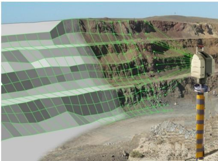
22 Сурет – Лазерлік - сканирлеу жүйелері
