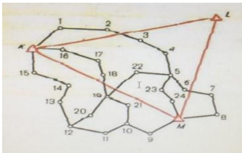
9 Сурет – Полигонометрия:
