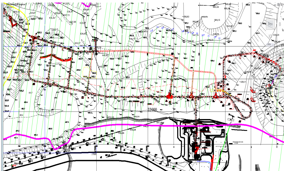
4 Сурет – Ақжал кенішіндегі тау-кен жұмыстарының жағдайы
