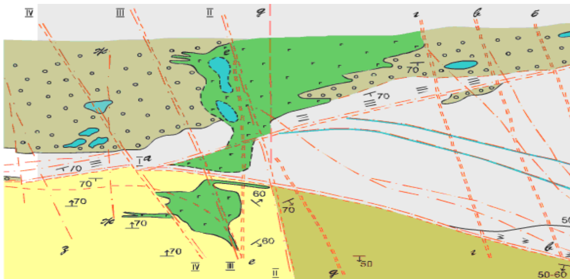
2 Сурет – Ақжал кен орнының тектоникалық картасы
